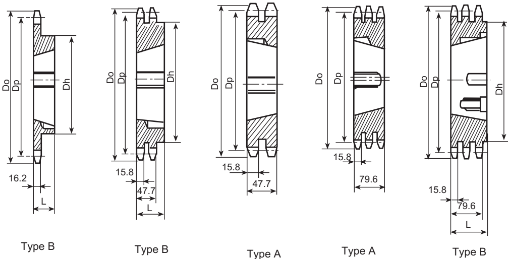
Taper Bored Sprockets Unit:mm
